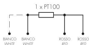
Schema connessioni
