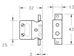
Femmina da pannello Female panel
