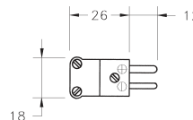
Femmina da pannello Female panel
