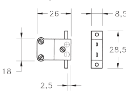
Femmina da pannello Female panel
